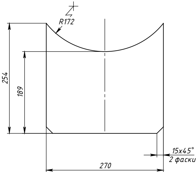
Поз.2 (Ребро)
